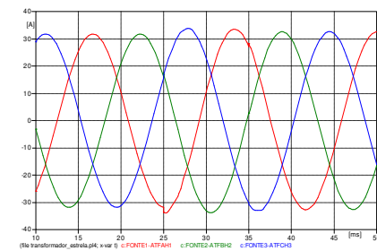
FIGURA 10.(a) – Corrente primária
