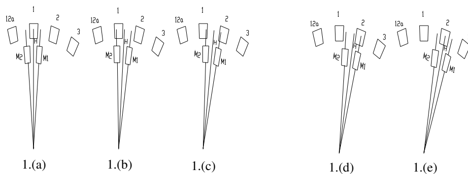
FIGURA 1 – Seqüência de chaveamento do seletor de derivação
