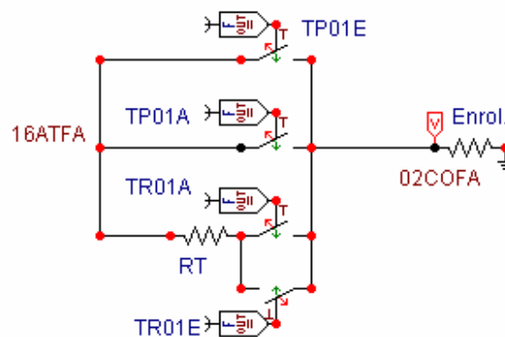
Figura 3 – Chaves controladoras conectadas ao enrolamento do transformador.
