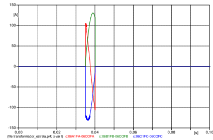
FIGURA 9.(d) – Corrente fechamento do tapresistor de transição.
