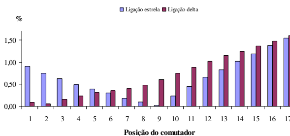
Figura 7 – Gráfico da diferença percentual da impedância de seqüência zero em modulo
