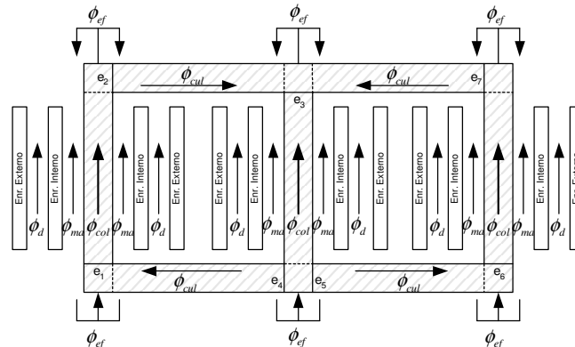
Figura 4 - Distribuição de fluxo fasorial num transformador trifásico de três colunas.
