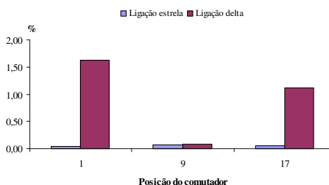
Figura 8 – Gráfico da diferença percentual da impedância de curto-circuito em modulo
