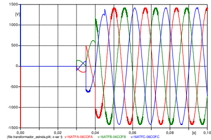
FIGURA 10.(b) – Comportamento da tensão no tap
