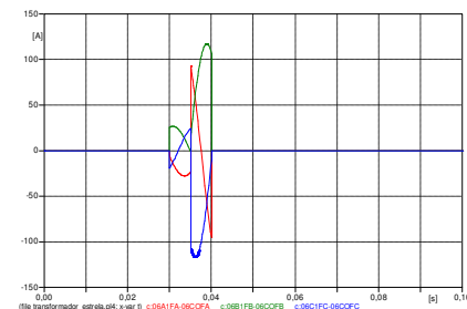
FIGURA 10.(d) – Corrente no resistor de transição
