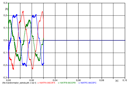
FIGURA 9.(c) – Corrente fechamento do tap.
