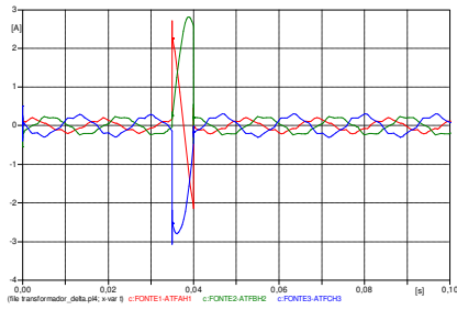
FIGURA 9.(a) – Corrente de magnetização
