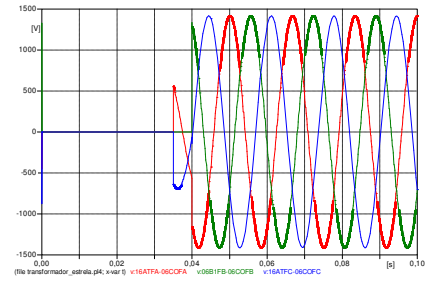
FIGURA 9.(b) – Comportamento da tensão no tap
