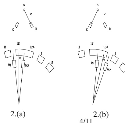
Figura 2 – Seqüência de chaveamento do seletor de comutação
