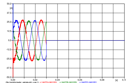
FIGURA 10.(c) – Corrente no fechamento do tap
