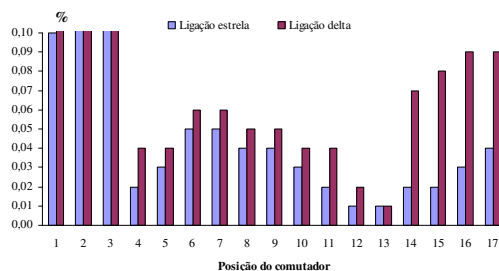
Figura 6 – Gráfico comparativo da diferença percentual da relação de transformação em modulo
