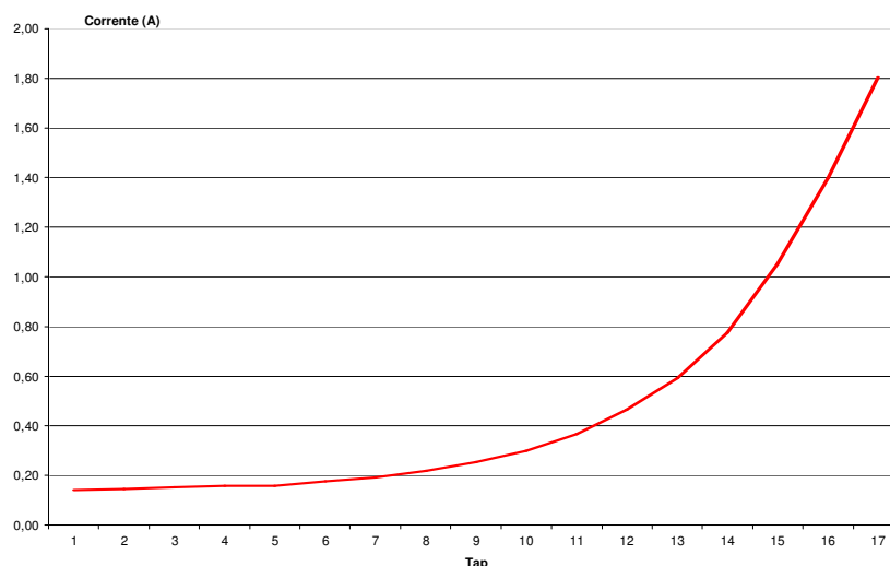
Figura 11 – Comportamento da corrente de magnetização tap a tap.
