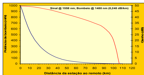
Figura 1. (a) Diagrama do sistema de transmissão sem repetição escolhido para a Eletronorte, onde L1 e L3 são as distâncias dos remotos até as estações terminais e L2 é a distância entre os remotos. (b) Gráfico da dependência da potência de bombeio e do ganho dos amplificadores remotos com a distância da estação.
