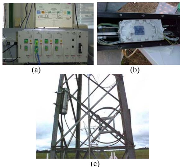
Figura 5 – (a) Sub-bastidor contendo as fontes de bombeio, o transponder bi-direcional, o pré-amplificador a fonte de alimentação e a placa de supervisão e controle na sub-estação Porto Velho, (b) Instalação do amplificador remoto na caixa de emenda óptica e (c) Caixa de emenda óptica com amplificador remoto instalada na torre de transmissão.
