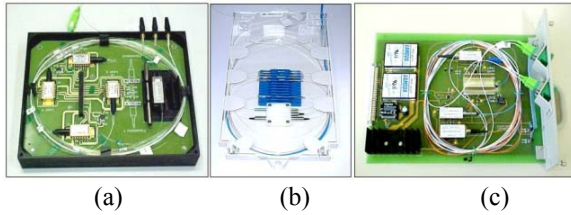
Figura 3 – (a) Fonte de bombeio, (b) Amplificador remoto no estojo de emenda e (c) Transponder bidirecional.
