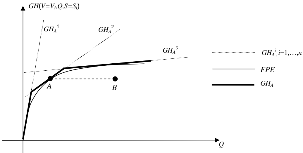
FIGURA 1 – Aproximação da FPE por planos tangentes para V e S constantes e três valores de Q
