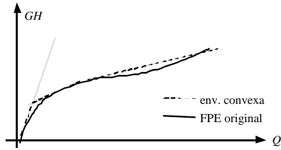
FIGURA 2 – Exemplo de construção da envoltória convexa para a região abaixo da FPE – corte nas dimensões Q e GH
