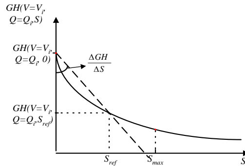
FIGURA 3 – Aproximação de GH na dimensão S
