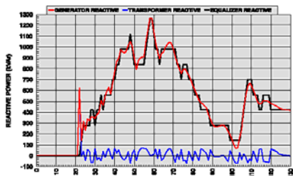
Figura 4- Medições de potências na partida
