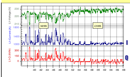
Figura 3 – Monitoração das variáveis elétricas antes e após a CRTR
