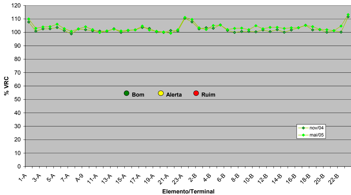
Figura 6: Medidas de Condutância – COS
