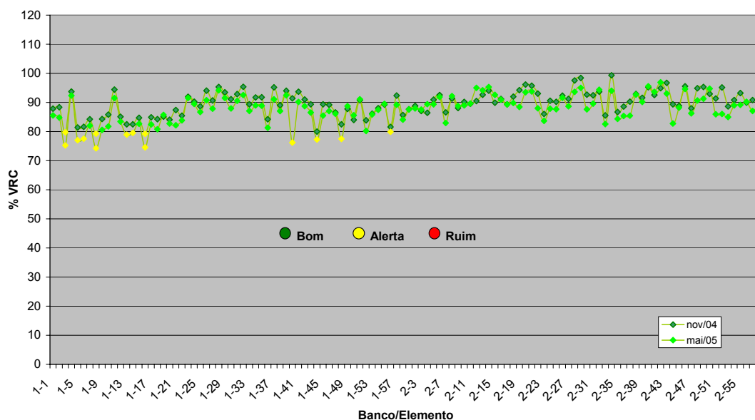
Figura 3: Medidas de Condutância – Subestação Pau Ferro
