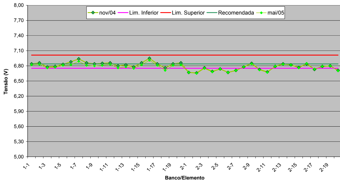
Figura 7: Medidas da Tensão de Flutuação – Mussuré Bancos 1 e 2
