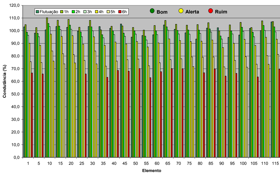
Figura 2: Condutância Durante a Descarga – Subestação Bongi
