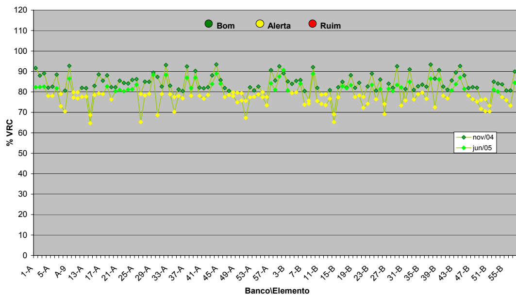
Figura 4: Medidas de Condutância – Luiz Gonzaga
