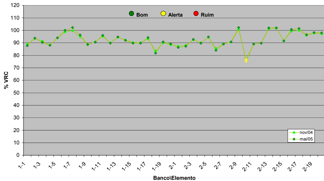
Figura 8: Medidas da Condutância – Mussuré Bancos 1 e 2
