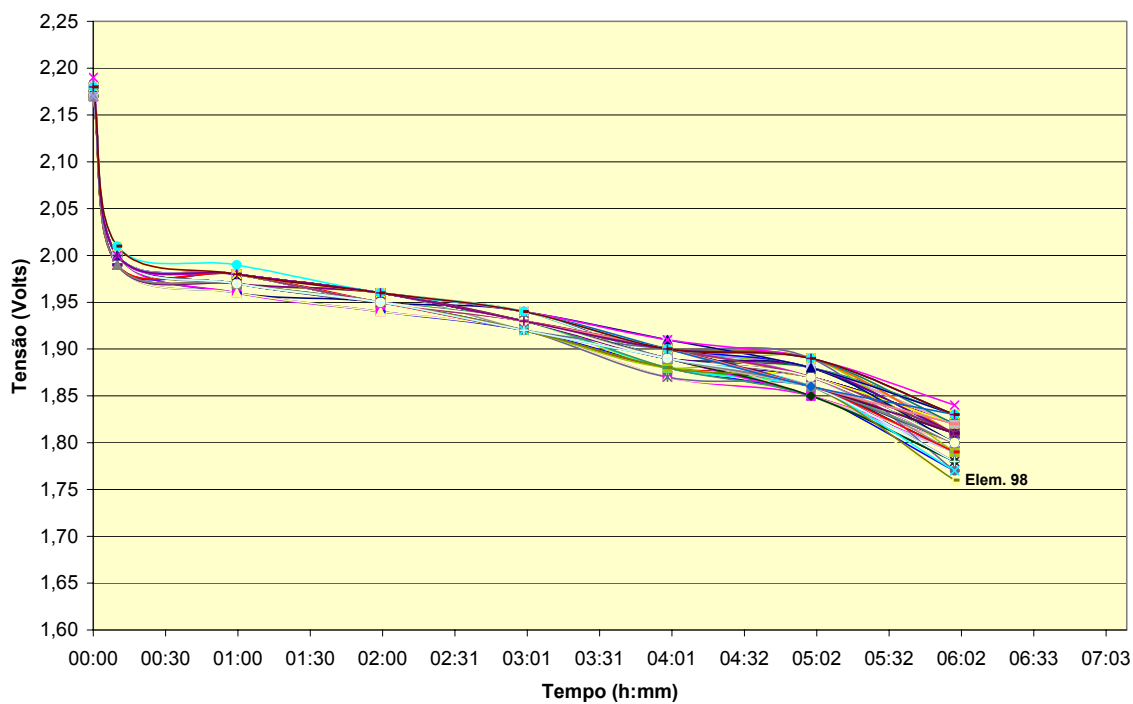
Figura 1: Teste de Capacidade - Subestação Bongi
