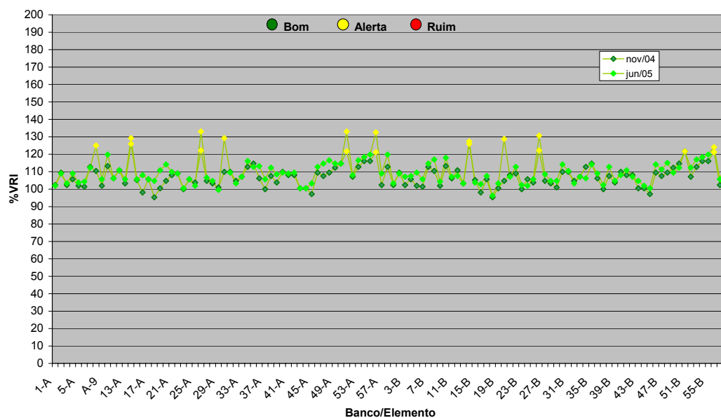
Figura 5: Medidas de Impedância – Luiz Gonzaga
