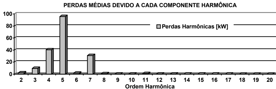
Figura 6 – Perdas Joulicas devido a cada componente harmônica
