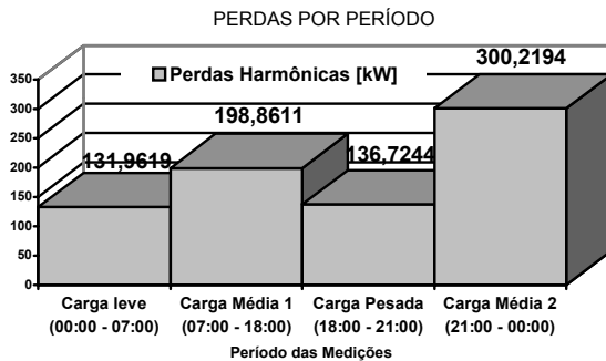
Figura 5. Perdas joulicas provocadas por um consumidor – média diária
