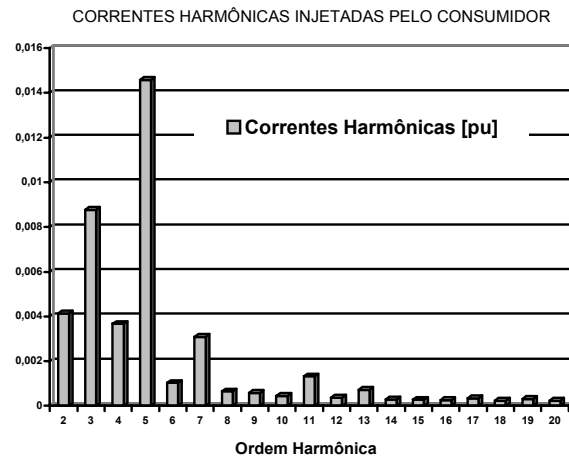
Figura 3. Correntes harmônicas injetadas por um grande consumidor.
