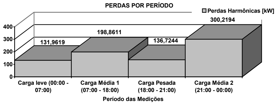
Figura 7 – Perdas ao longo de 24 Horas
