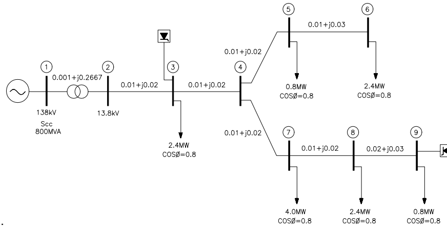
Figura 2. Sistema de 9 barras
