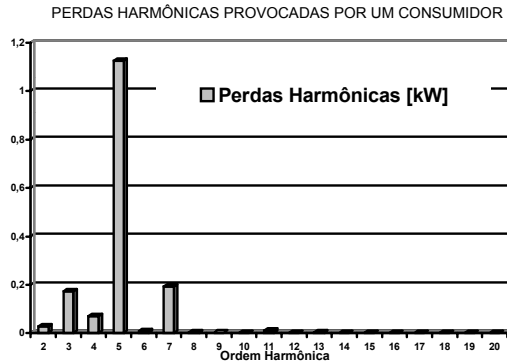
Figura 4. Perdas joulicas por harmônicas em todo o sistema devido a um grande consumidor
