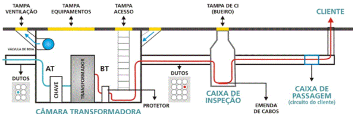
FIGURA 1 – Componentes do sistema subterrâneo
