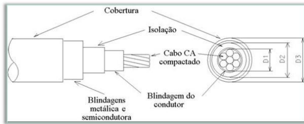
Figura 1 : Esquema de isolamento do cabo isolado
