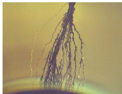
Fotos 5 e 6 : Fotos microscópicas de descargas em arborescência elétrica
