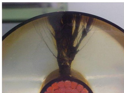
Fotos 5 e 6 : Fotos microscópicas de descargas em arborescência elétrica
