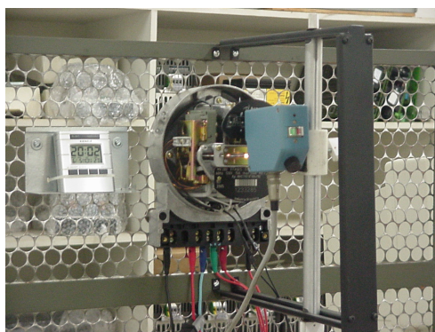
Figura 4 – Sensor de voltas de disco acoplado a medidor bifásico do tipo indução em teste.
