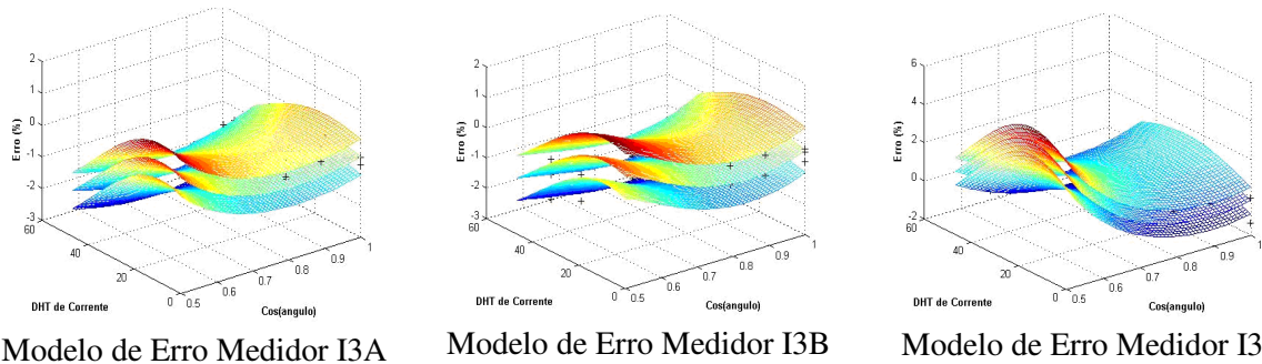
Figura 9 – Superfícies dos Modelos de erro de medição encontradas para três amostras de diferentes medidores de energia do tipo indução trifásicos, considerando desequilíbrio de tensão de 3%.
