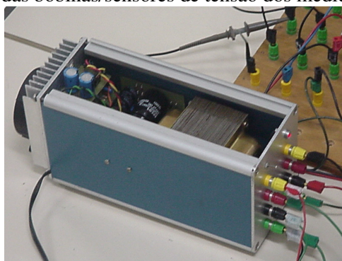
Figura 3 – Amplificador de tensão CA trifásico desenvolvido.
