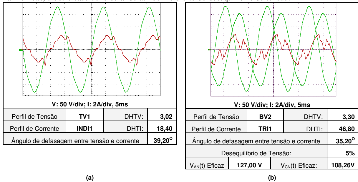
Figura 6– Exemplos dos perfis de tensão e corrente utilizados nos ensaios experimentais: (a) considerando somente distorção harmônica (b) considerando distorção harmônica e desequilíbrio de tensão.
