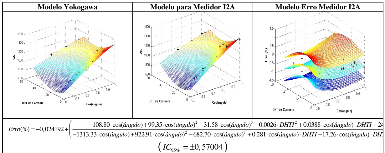
Figura 8– Superfícies dos modelos encontrados para a amostra I2A dos medidores de energia do tipo indução bifásico, e a expressão do erro de medição sem considerar condições de desequilíbrio de tensão.
