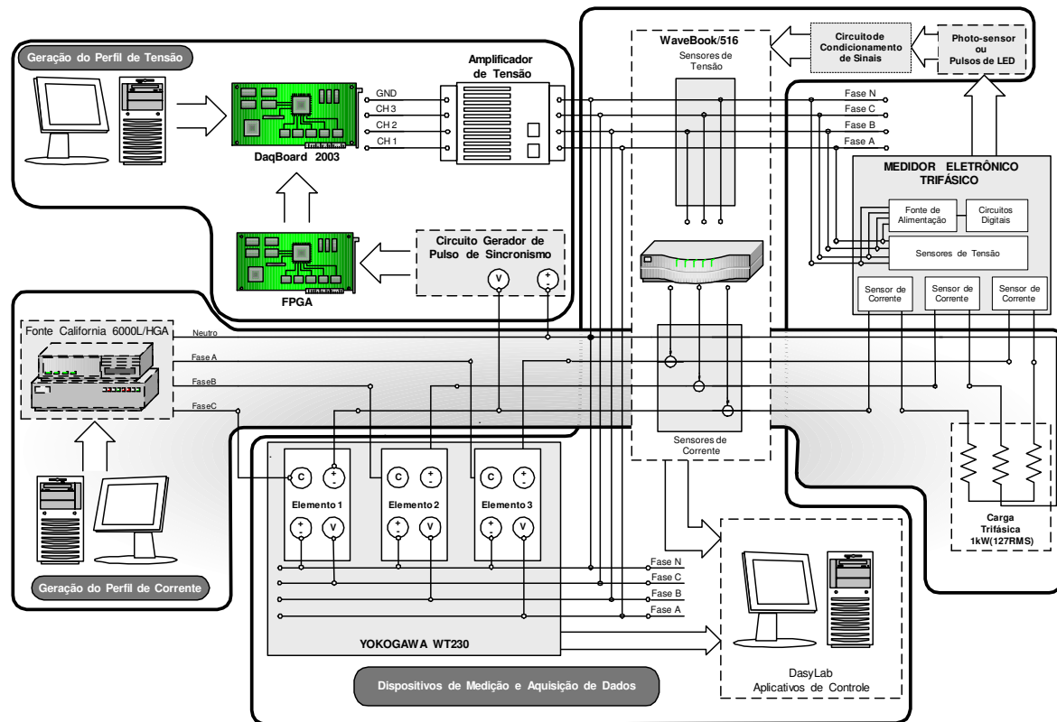
Figura 1 - Diagrama de blocos do sistema proposto, exemplo da configuração utilizada na avaliação dos medidores trifásicos eletrônicos.
