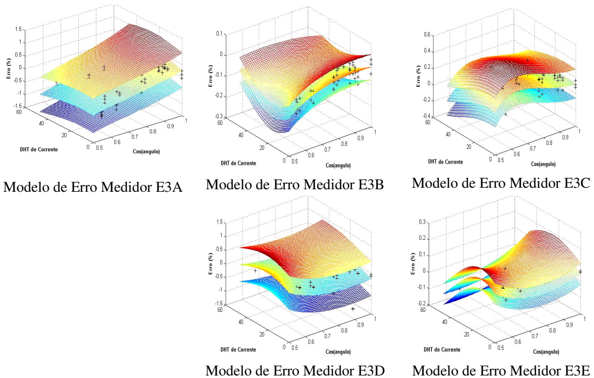
Figura 10 – Superfícies dos Modelos de erro de medição encontradas para as cinco amostras de medidores de energia do tipo eletrônicos trifásicos, sem considerar desequilíbrio de tensão.
