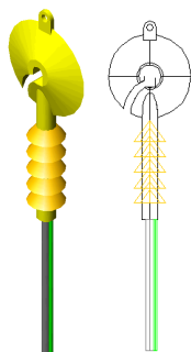
Figura 5 – Primeiro esboço de um design da sonda
