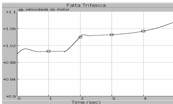
Figura 7 – Velocidade de uma unidade geradora
