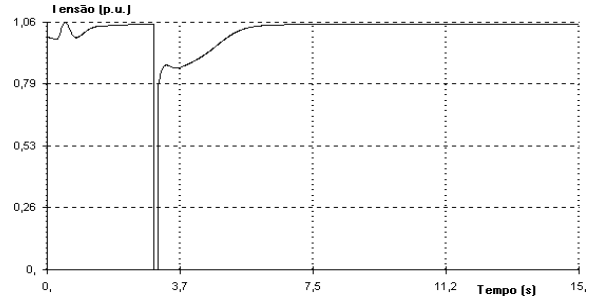
Figura 3 – Tensão (em p.u.) em Brumado no tempo (s)
