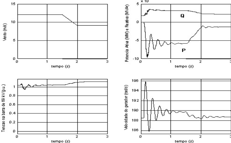
Figura 5 – Conexão da Usina em vento nominal e decrescimento do vento.
