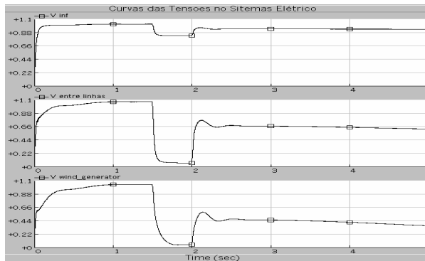
Figura 6 – Tensões nas diversas barras
