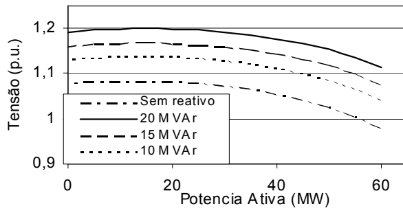
Figura 2 – Perfil de tensão em Caetité para diversos níveis de compensação local de reativos
