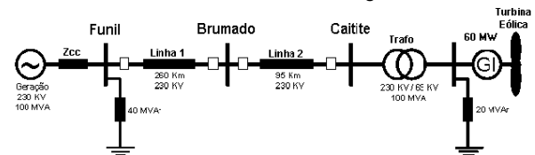
Figura 1 – Arranjo básico do sistema elétrico
