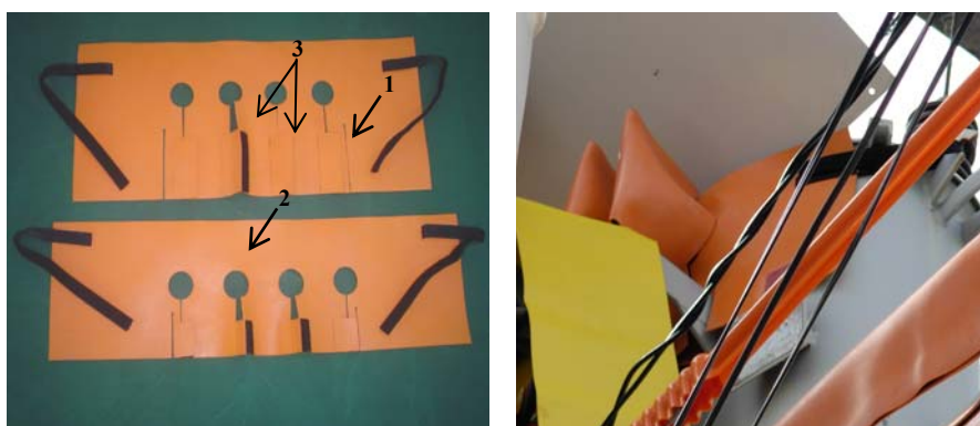
FIG. 10 – LENÇÓIS ISOLANTES PARA O TANQUE (1), SUPORTE (2) E TERMINAIS SECUNDÁRIOS DO TRANSFORMADOR (3)
