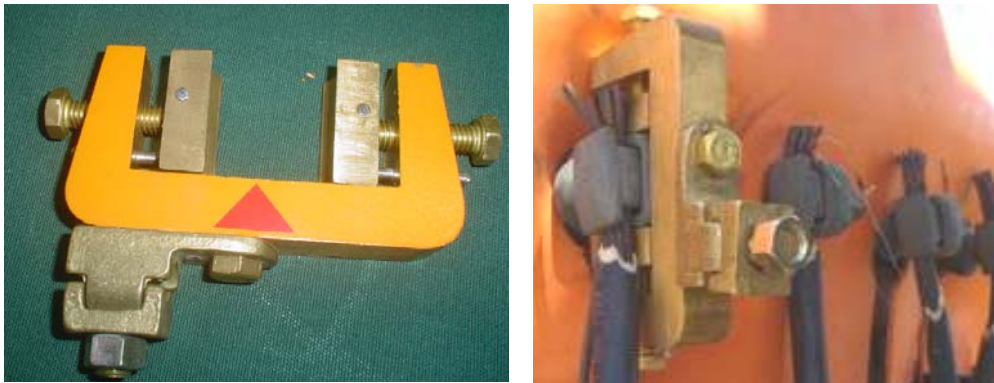
FIG. 8 – DISPOSITIVO DE ACOPLAMENTO DAS BUCHAS DE BAIXA TENSÃO, PARA CORRENTES DE ATÉ 400 A
