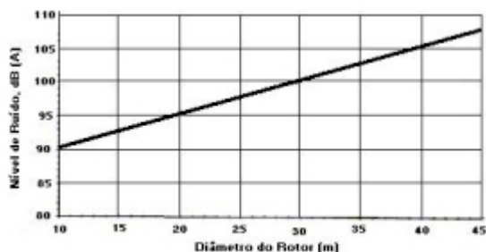
FIGURA 3 - Nível de ruído para diversas turbinas eólicas disponíveis em 1995.
