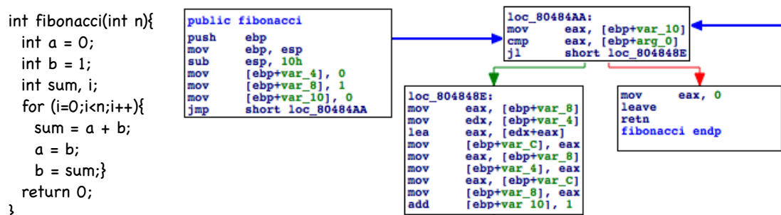
Figura 1. Programa em linguagem C e o grafo de fluxo correspondente.
